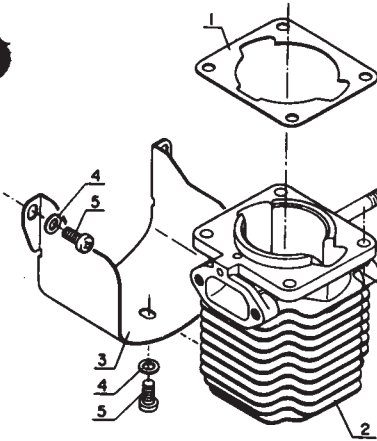
— CYLINDRE ET ECHAPPEMENT —
