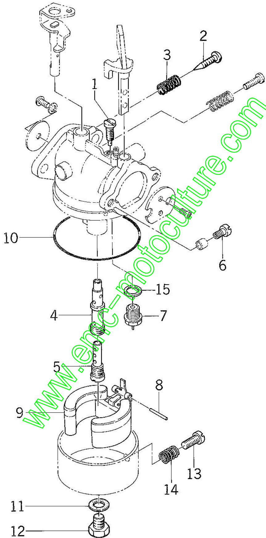
Fig. 4A CARBURETOR (for KF522-A) Carburateur (pour KF522-A)
