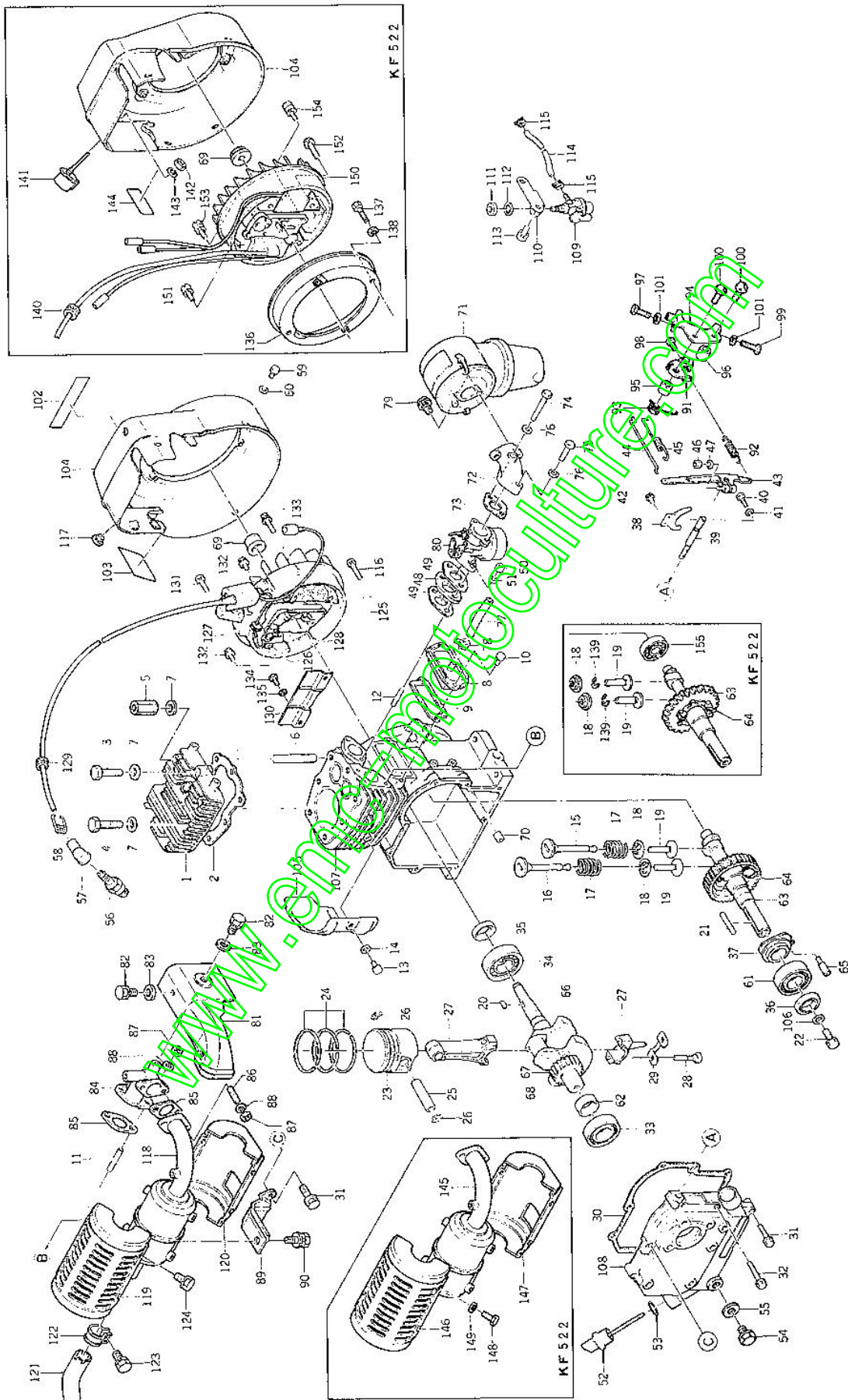
Fig. 1 ENGINE (KF522-A, KF522) Moteur (KF522-A, KF522)
