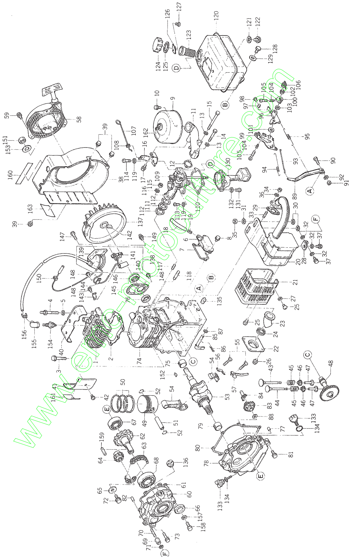
Fig. E-1 ENGINE (FA130G-12 314419A) Moteur
