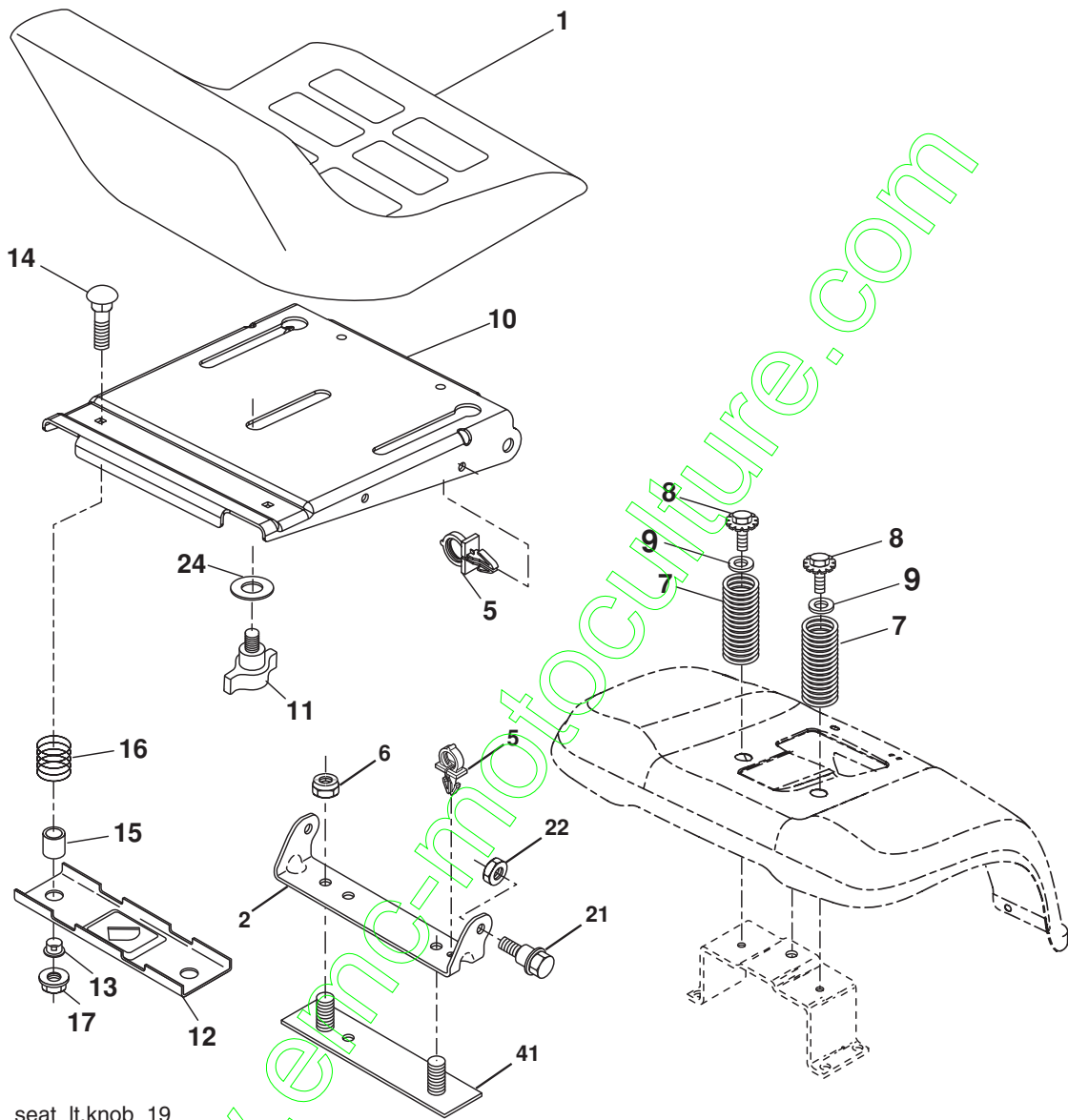
seat_lt.knob_19
