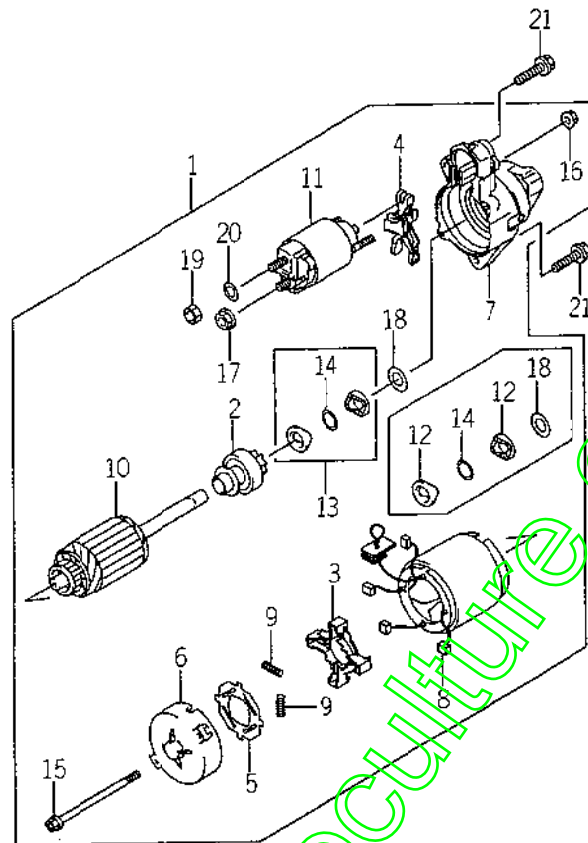
FIG. 11 STARTER
