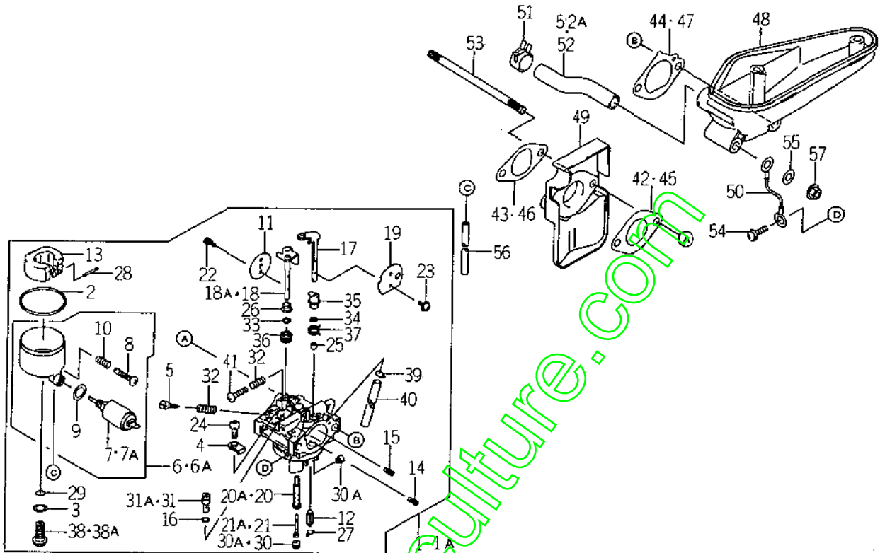
FIG. 8 CARBURETOR
