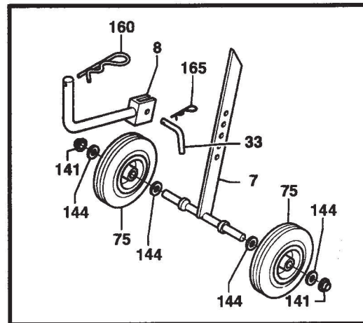
18501300 KIT ROUES DE TRANSPORT
